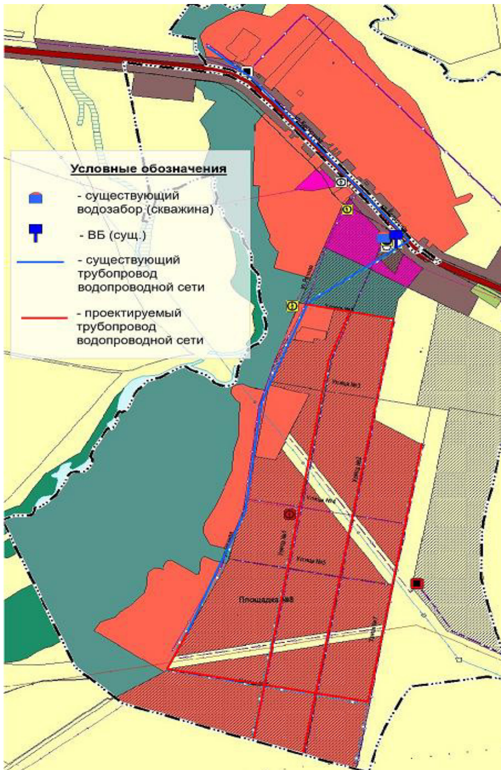
Рисунок 2.4.9.3– Схема существующего и планируемого размещения объектов централизованной системы водоснабжения в с. Нижняя Козловка
