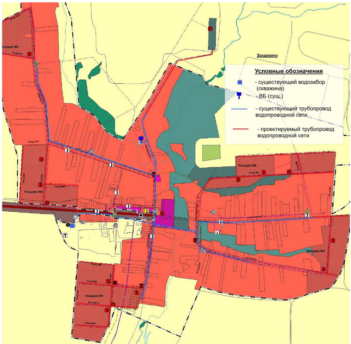
Рисунок 2.4.9.1– Схема существующего и планируемого размещения объектов централизованной системы водоснабжения в с. Захаркино
