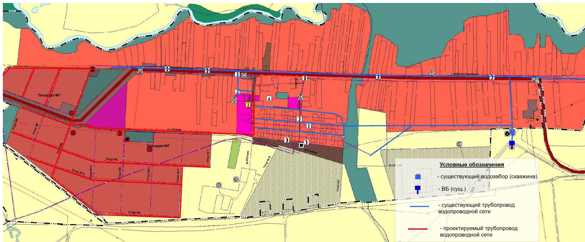
Рисунок 2.4.9.2 – Схема существующего и планируемого размещения объектов централизованной системы водоснабжения в с. Сидоровка
