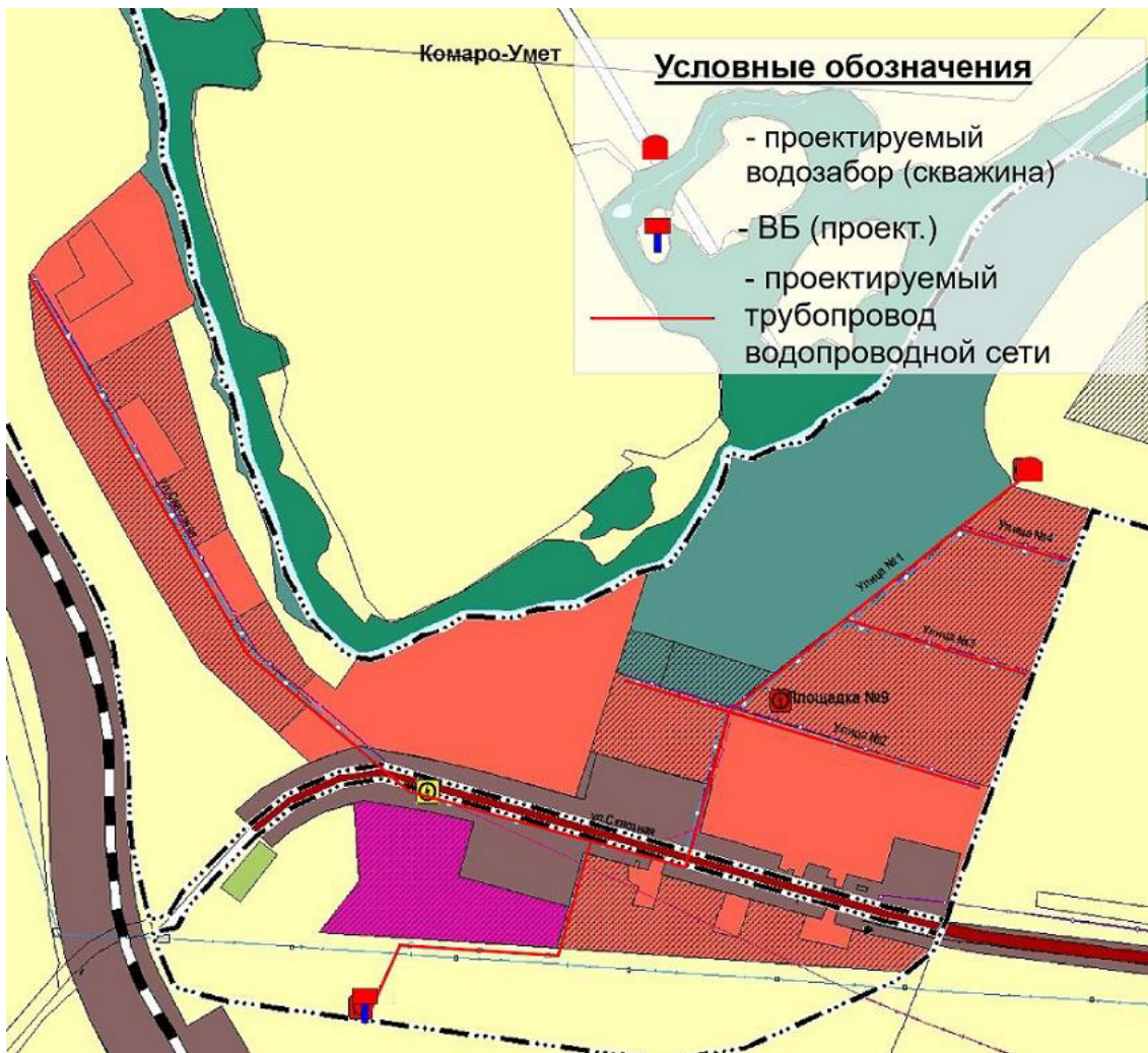
Рисунок 2.4.9.4 – Схема существующего и планируемого размещения объектов централизованной системы водоснабжения в с. Комаро-Умет
